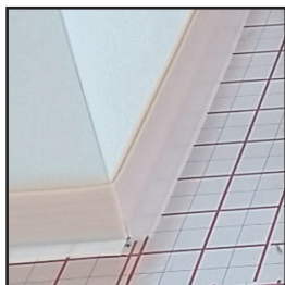
Perfekte strakke aansluitingen met Redumax Kantstrook DUO® met zelfverende voet en haaksehoek technologie klaar om vloeistofdicht te worden afgetaped met Redumax Tape®.
