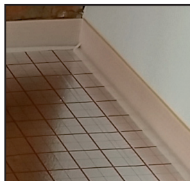
Perfekte strakke aansluitingen met Redumax Kantstrook DUO® met zelfverende voet en haaksehoek technologie klaar om vloeistofdicht te worden afgetaped met Redumax Tape®.
